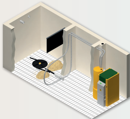
KWB Pilleomrører Plus med sugetransport
