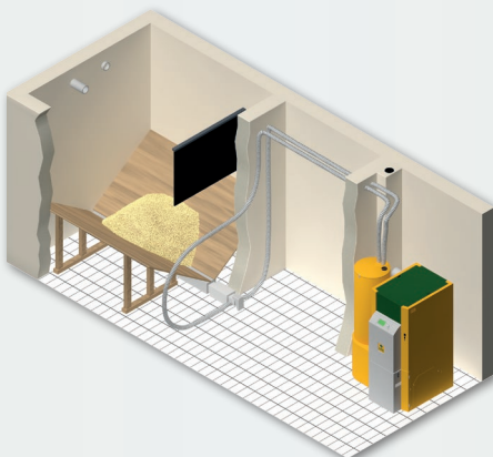
Transportsnegl med sugetransport
