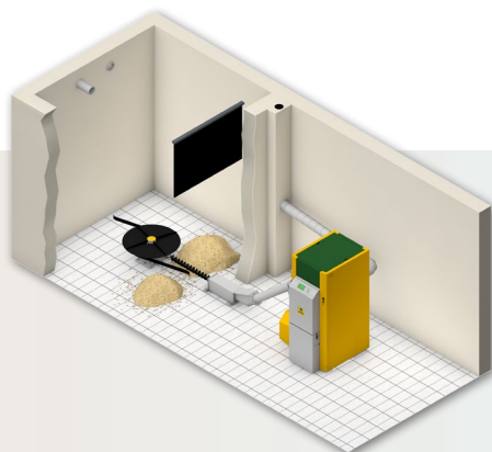
KWB Pilleomrører Plus med knæksnegl
