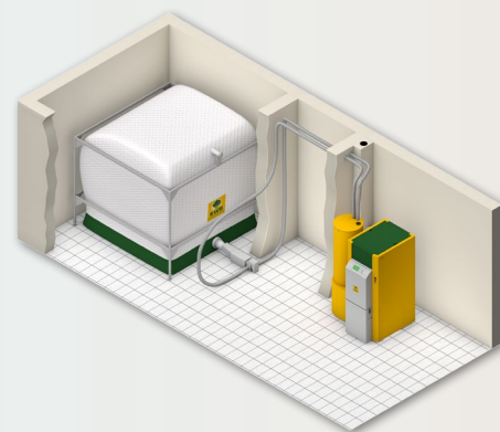
KWB Pellet Big Bag med sugetransport
