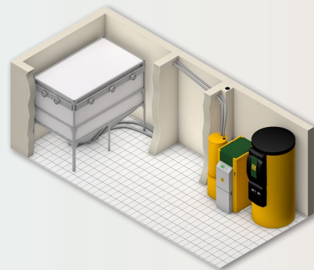
KWB Pellet Box med sugetransport
