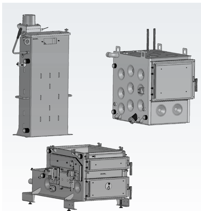
KWB Classicfire – kedel kan adskilles i 3 dele
